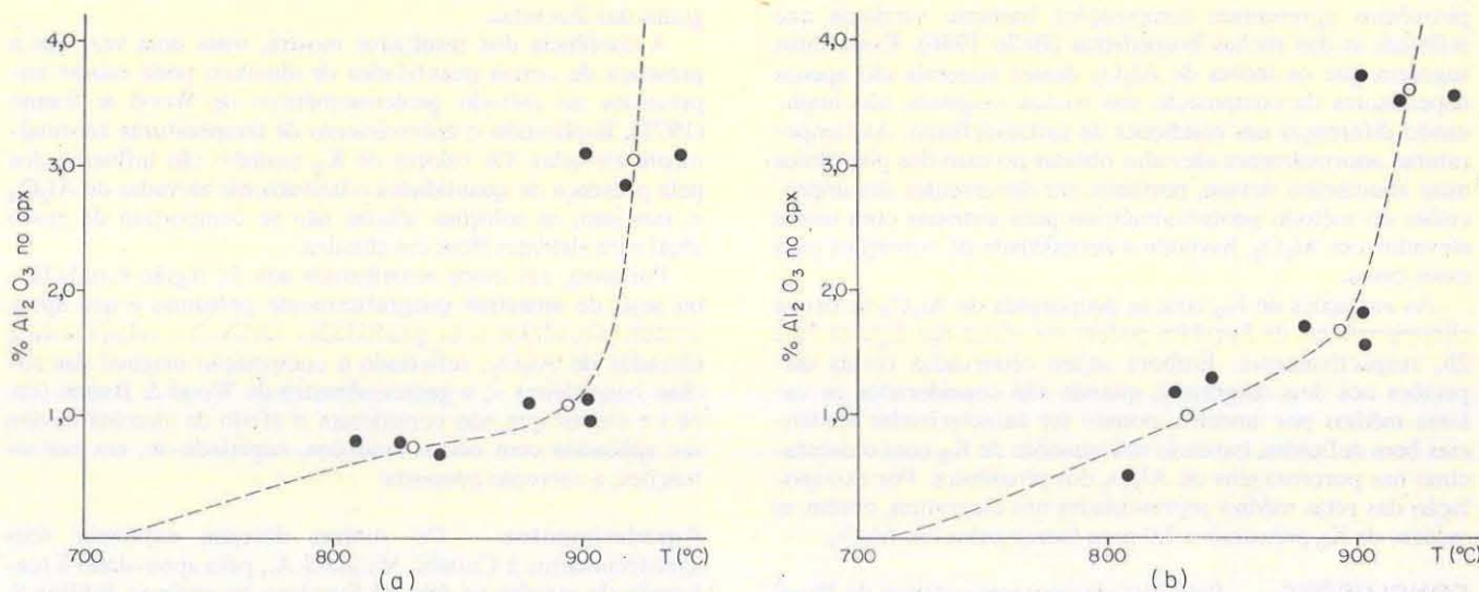
Figura 1 - Correlações entre as porcentagens em peso de Al 2 O 3 dos ortopiroxênios (a) e clinopiroxênios (b) de Surubim e as temperaturas obtidas pelo método de Wood & Banno (1973). Círculos cheios: valores obtidos a partir de cristais individuais de cada amostra; círculos vazios: valores determinados pela média por amostra
